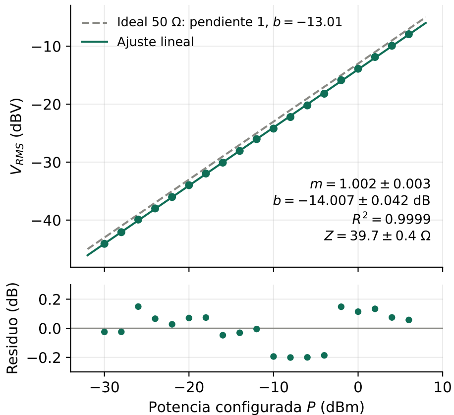
(b) Escala en dB: relación lineal
