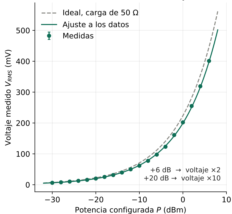
(a) Escala lineal: crecimiento exponencial
